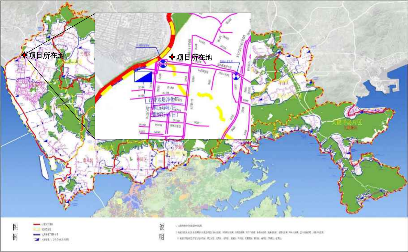
附图 13 项目所在区域污水管网图
